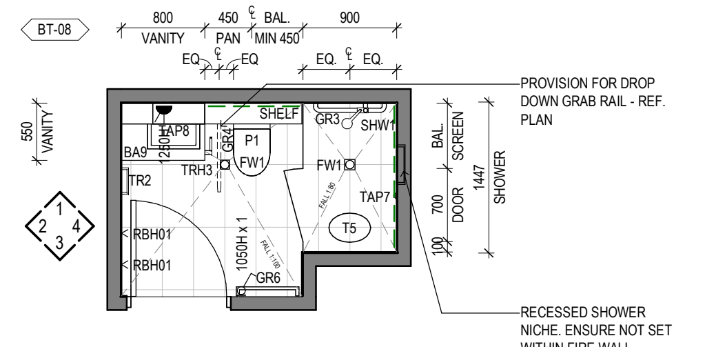
3 ILA BT-08 Scale 1 : 50
