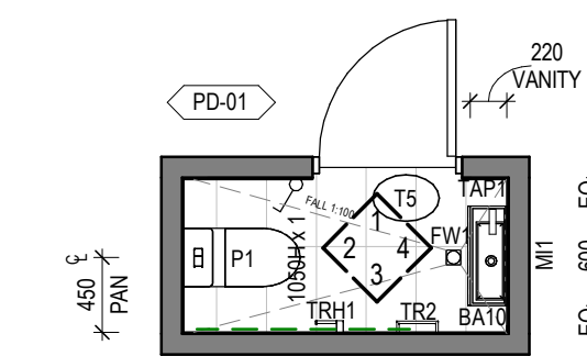
5 ILA PD-01 Scale 1 : 50
