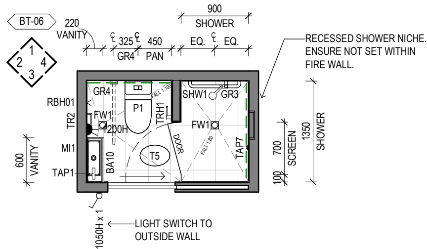
1 ILA BT-06 Scale 1 : 50
