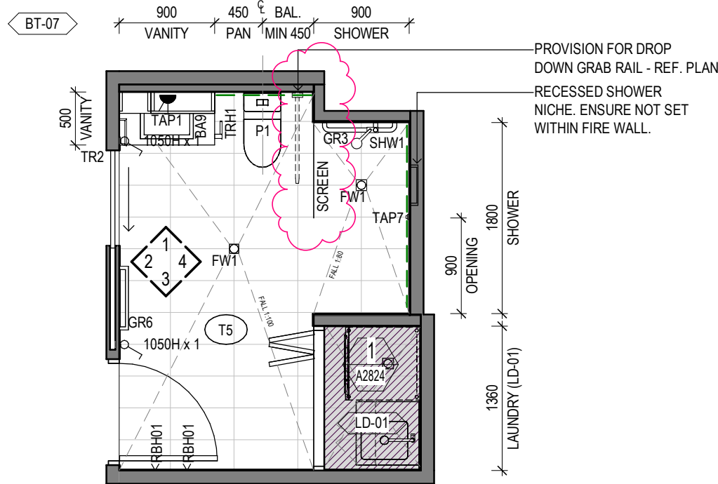
2 ILA BT-07 Scale 1 : 50
